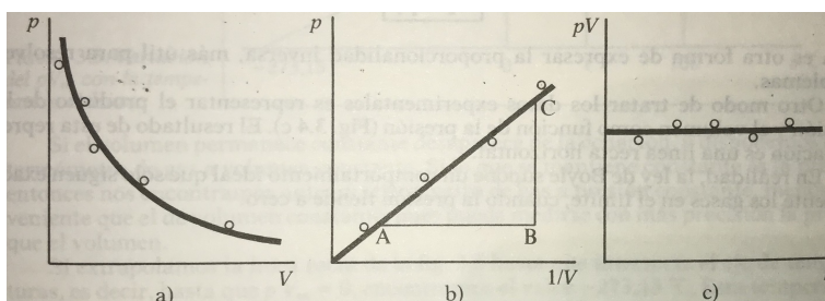
Figura 1.2: Experiment de Boyle i llei de proporcionalitat entre la pressió exercida sobre un gas i el seu volum.
