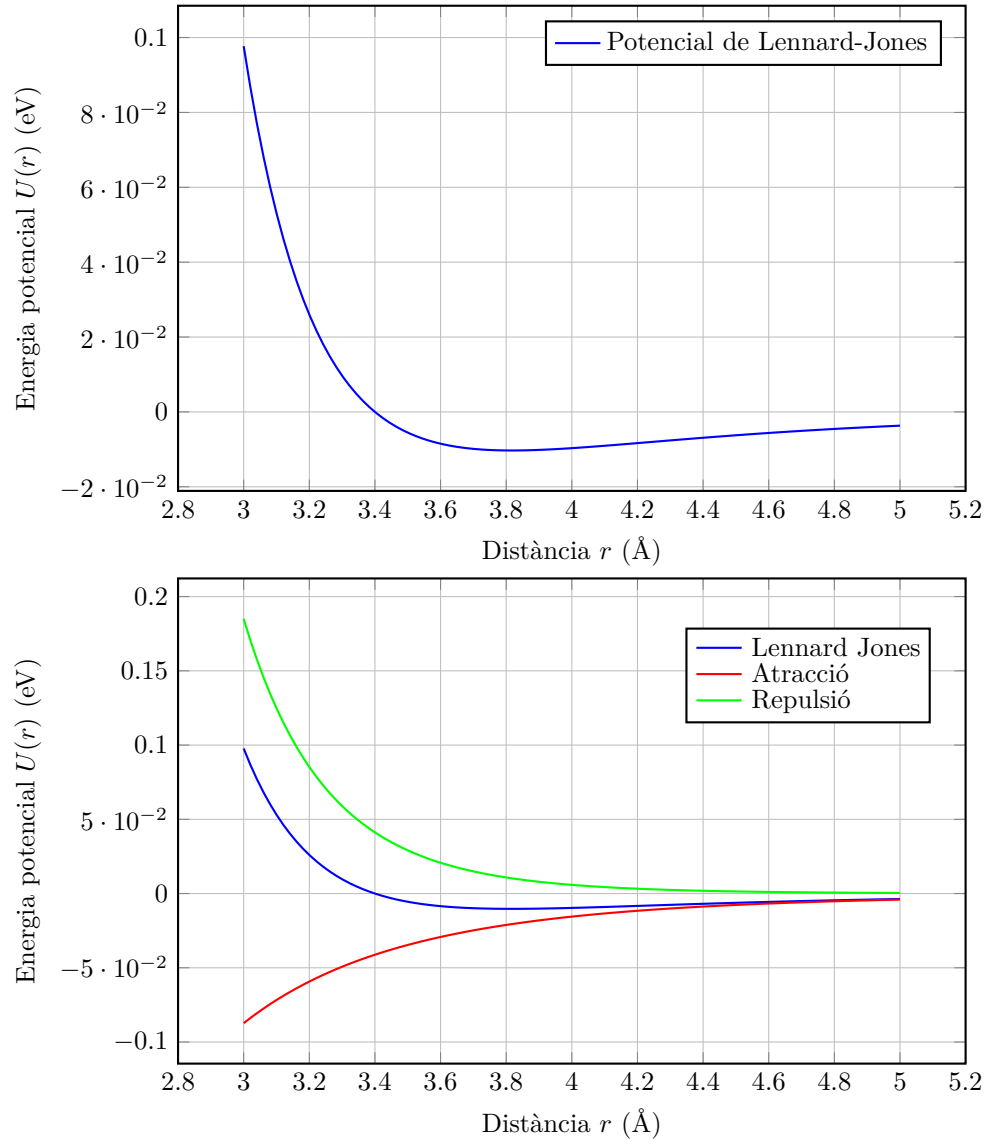
Figura 1.8: Potencial de Lennard-Jones amb valors típics ( \varepsilon = 0,010 eV, \sigma = 3,4 Å). L'energia potencial disminueix inicialment fins a un mínim, corresponent a la distància d'equilibri on la interacció és més estable. Quan les molècules s'acosten massa, la repulsió electrònica domina i l'energia potencial augmenta ràpidament.
