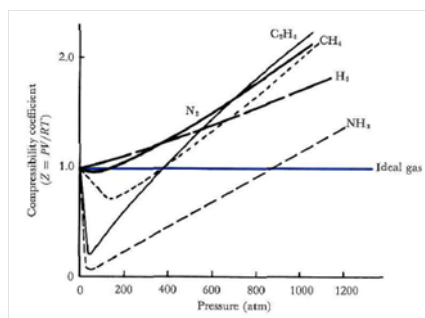
Figura 1.4: R es pren com al valor límit de la fracció \frac{PV_m}{T} per a tots els gasos: R = \lim_{P \rightarrow 0} \frac{PV_m}{T} = 0.08205 \frac{\text{atm l}}{\text{mol K}}
