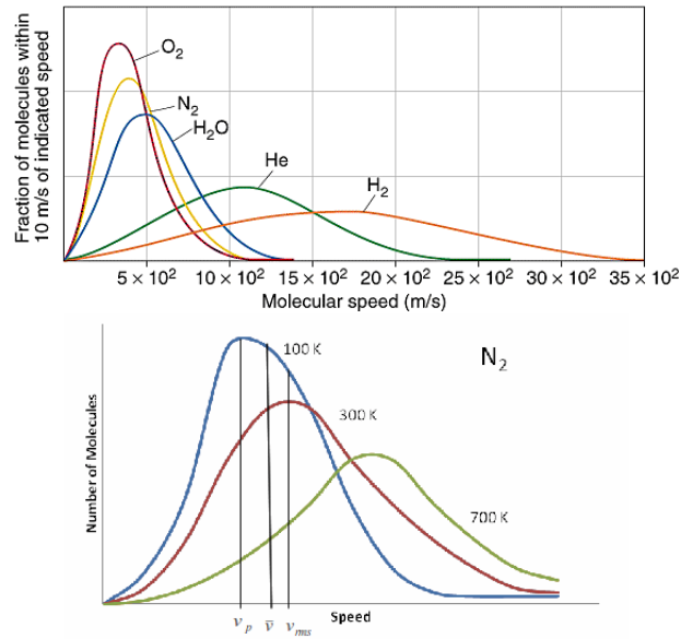
Figura 1.6: La distribució de Maxwell-Boltzmann per a diferents molècules i temperatures
