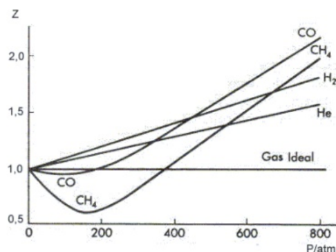
Figura 1.7: Factor de compressibilitat per a diferents gasos a 0°C.
