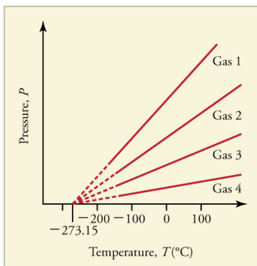
Figura 1.3: Gràfic del zero absolut a partir de la llei de Charles i Gay-Lussac.
