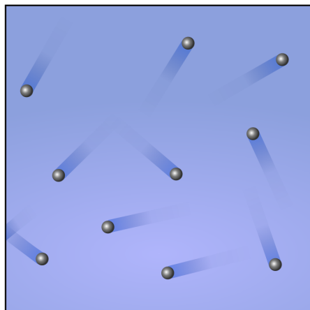
Figura 1.5: Representació del moviment de les partícules en un gas ideal.
