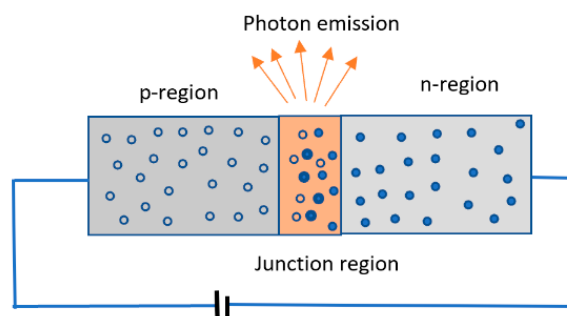
(a) Esquema d'un LED.
