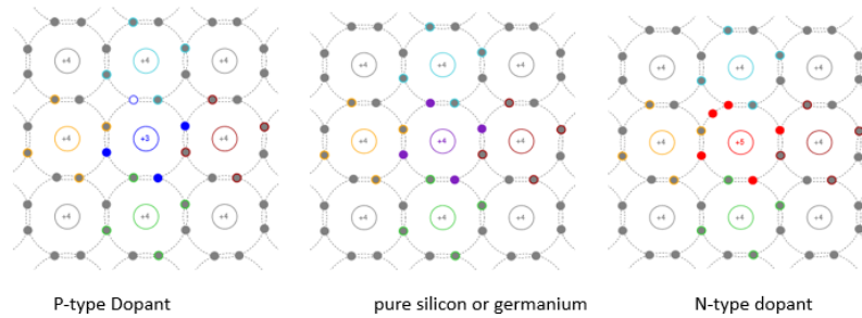
Figura 7.22: Els díodes es poden fabricar dopant elements com el silici i el germani (que típicament tenen 4 electrons de valència) amb elements de mida similar que tenen 3 o 5 electrons de valència; els primers creen la capa P i els segons la capa N.
