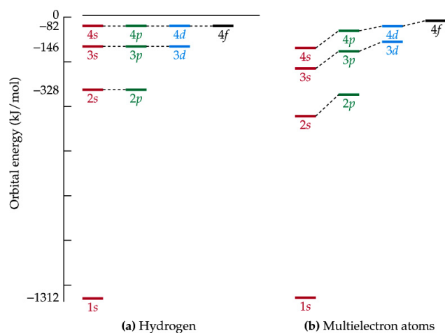
Figura 7.14: Degeneració dels orbitals de l'àtom d'hidrogen i d'àtoms polieletrònics
