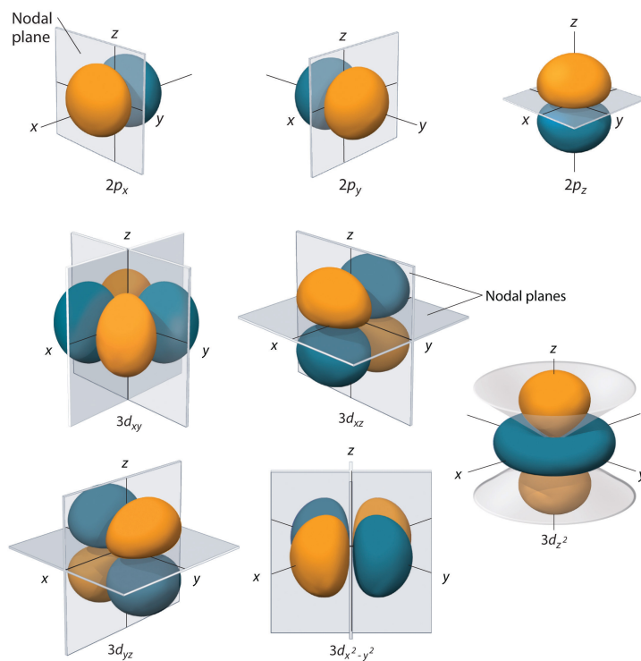
Figura 7.13: Densitat electrònica dels orbitals 2p i 3d de l'hidrogen. Font: Chem Libretext
