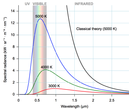
Figura 7.3: Distribució de freqüències de radiació emeses per un cos negre
