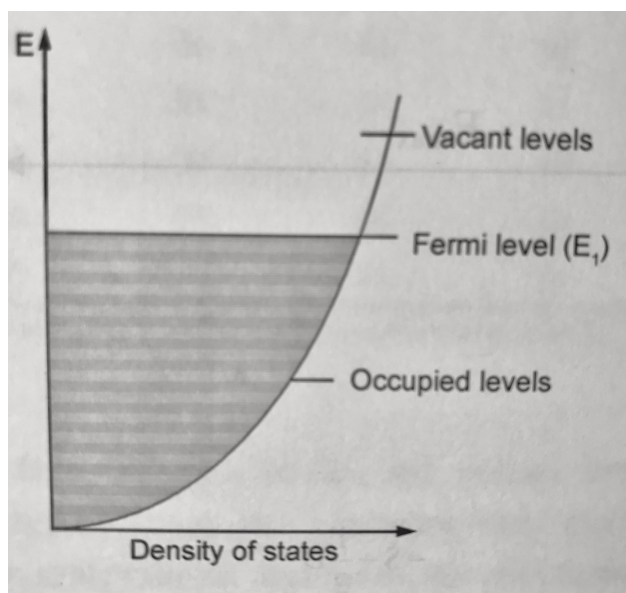
Figura 7.20: En el model de l'electró lliure, la densitat d'estats d'un gas d'electrons és proporcional a l'arrel quadrada de l'energia cinètica de les partícules [5].
