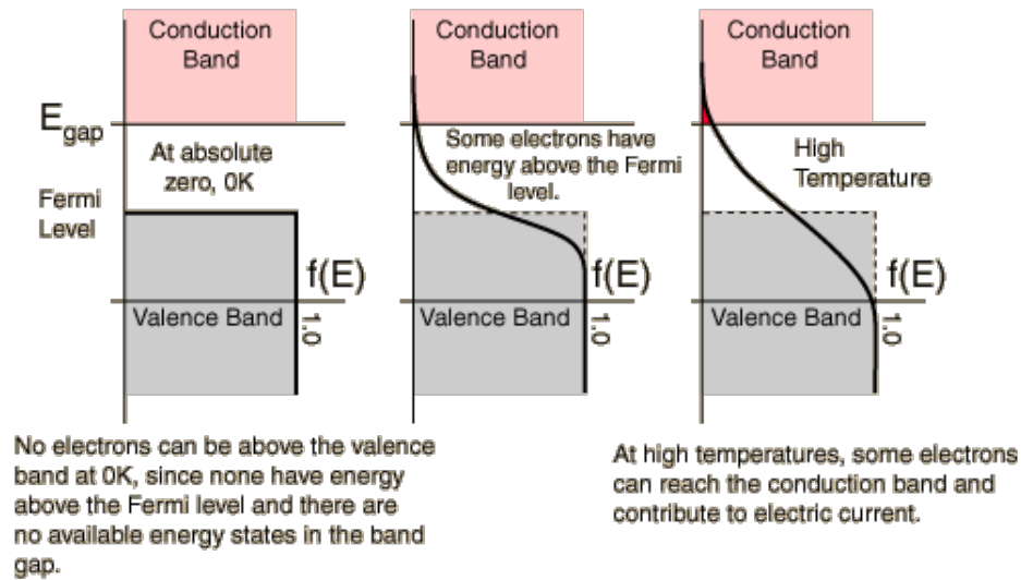
Figura 7.19: Efecte de la temperatura en un semiconductor.
