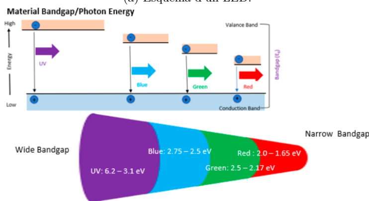
(b) Bretxa de banda de la llum UV, blava, verda i vermella.
