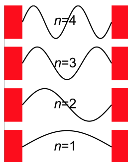
Figura 7.11: Funcions d'ona corresponents als primers nivells d'energia d'una partícula en una caixa unidimensional.
