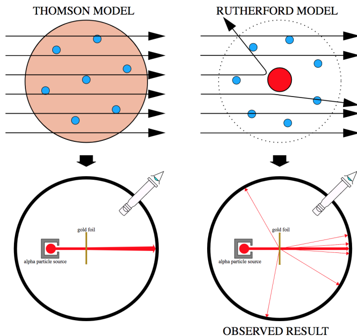
Figura 7.7: La figura de l'esquerra mostra com haurien de travessar una placa metàl·lica partícules \alpha segons el model de Thomson, A la dreta de la figura apareix l'explicació del comportament experimental real segons el model de Rutherford.
