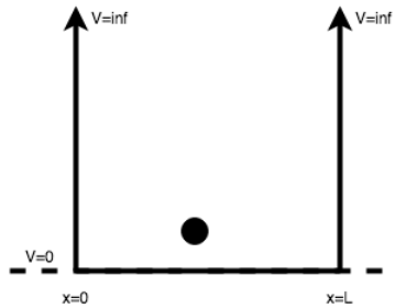
Figura 7.10: Partícula en una caixa unidimensional de potencial V = 0 entre x = 0 i x = L i V = \infty en qualsevol altre posició
