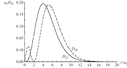
(b) Funció de distribució radial D(r) per a les funcions 2s i 2p
