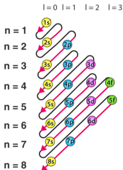
Figura 7.16: Ordre d'ompliment dels orbitals segons el principi d'Aufbau
