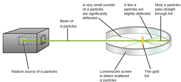
Figura 7.6: L'experiment de Rutherford.
