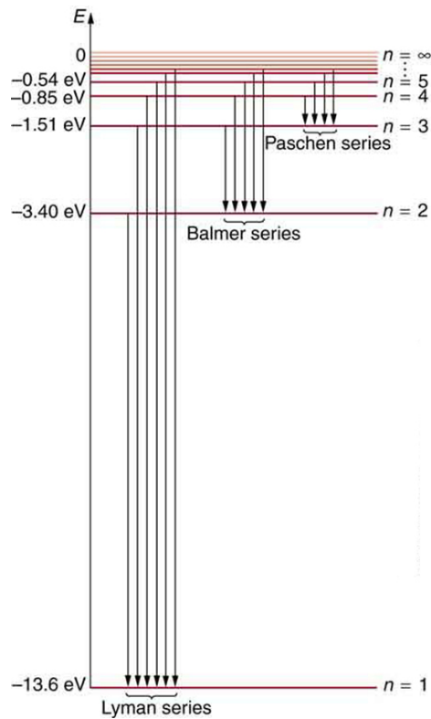
Figura 7.9: Diagrama de nivells d'energia per a l'hidrogen mostrant les sèries de Lyman, Balmer i Paschen de transicions. Les energies orbitals es calculen utilitzant l'equació anterior, derivada per primer cop per Bohr.
