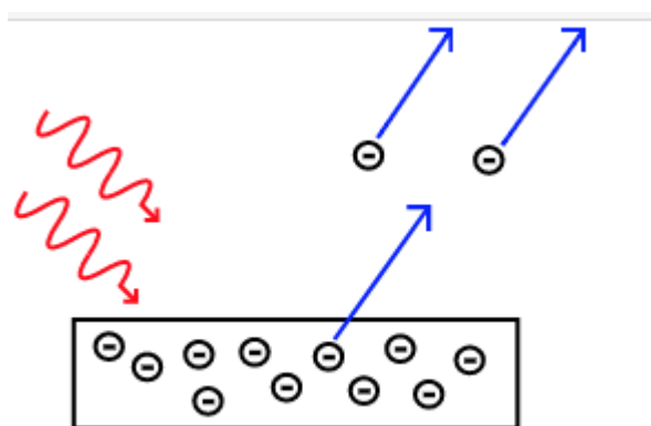
Figura 7.4: Efecte fotoelèctric
