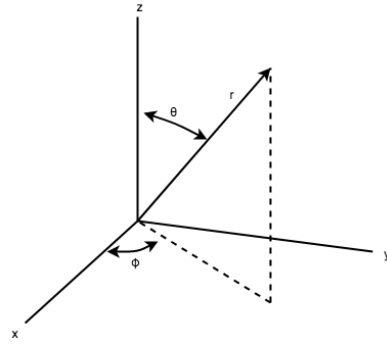
(a) Coordenades esfèriques.
