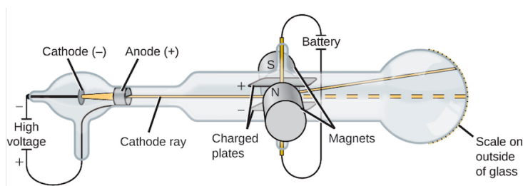
Figura 7.5: Un diagrama del tub de raigs catòdics de J.J. Thomson. El raig s'origina al càtode i passa a través d'una esclatxa a l'ànode. El raig catòdic es desvia lluny de la placa elèctrica carregada negativament i cap a la placa elèctrica carregada positivament. La quantitat amb què el raig es desviava per un camp magnètic va ajudar Thomson a determinar la relació massa-càrrega de les partícules. Font: Khan academy
