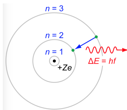
Figura 7.8: Model de l'àtom de Bohr
